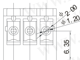
A 向视图
