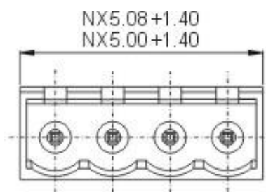
2EDGVC-5.0 2EDGVC-5.08
