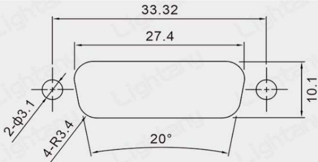
3V3机箱面板开孔尺寸
