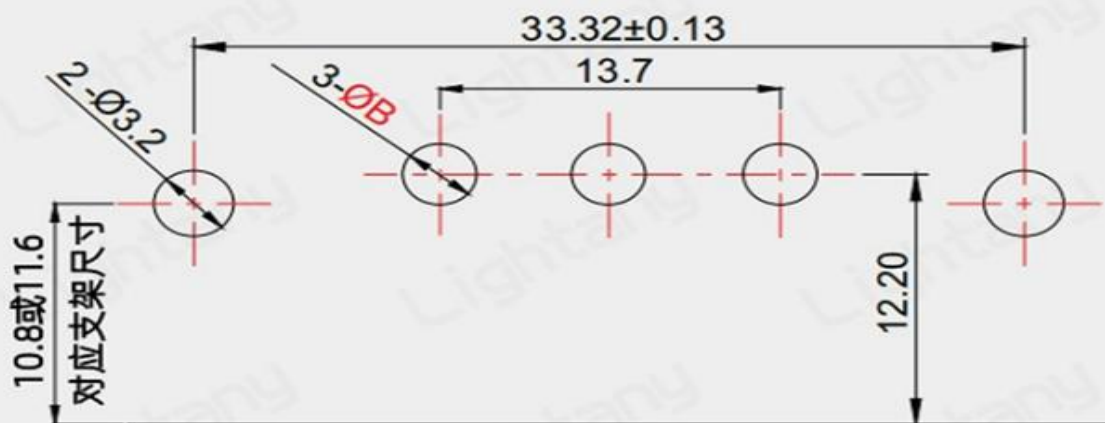
直插板PCB板开孔尺寸
