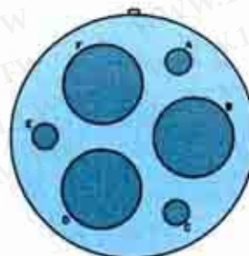
36-3 3-#12 3-#0 D
