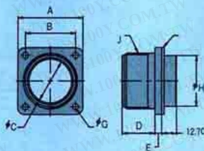
MS 3102 可安裝在機箱的插座 Box Mounting Receptacle
