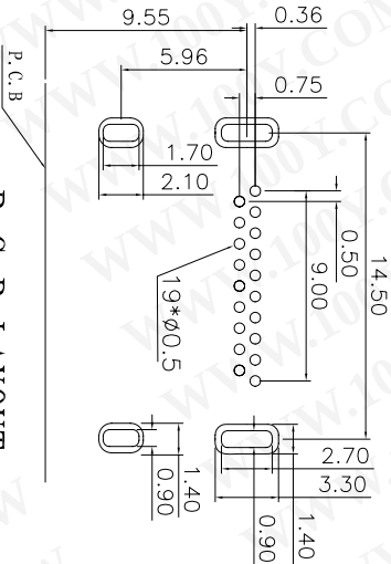
P.C.B LAYOUT
