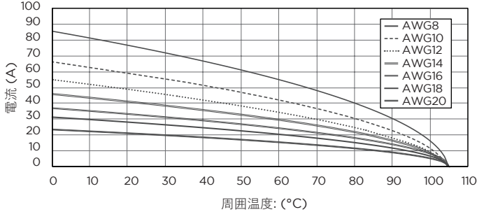
温度上昇曲線
