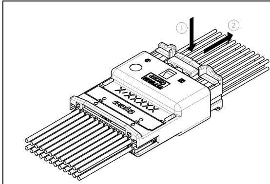
Fig.26 Déflexion du linguet Deflexion of locking lance
