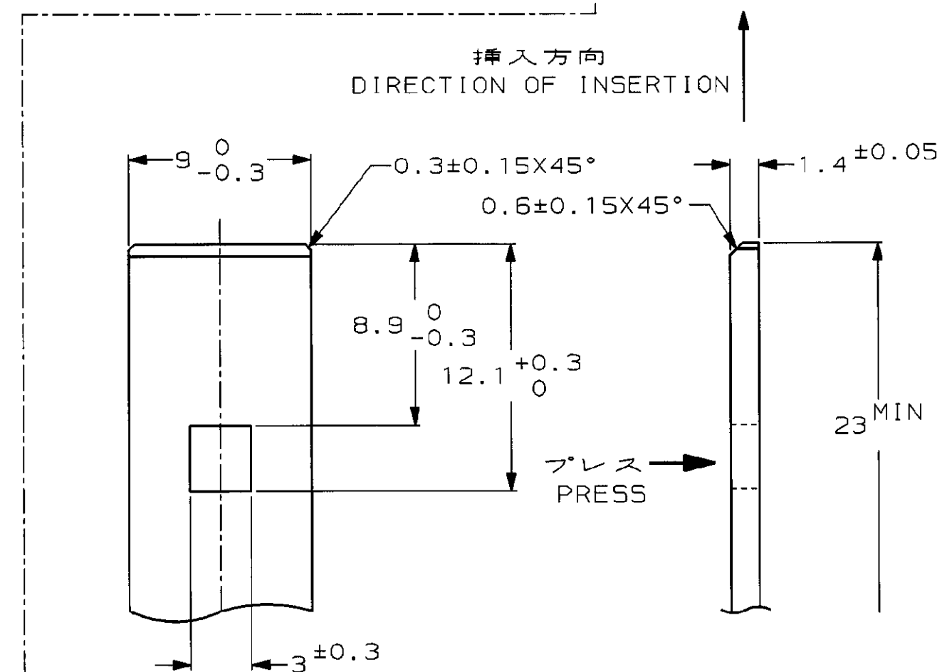
ブラケット推奨寸法図 RECOMMENDED DIMENSIONS OF BRACKET SCALE 4 : 1
