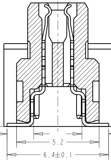
SECT "A" - "A" (SCALE: 8-1)
