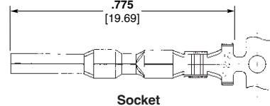
Socket
