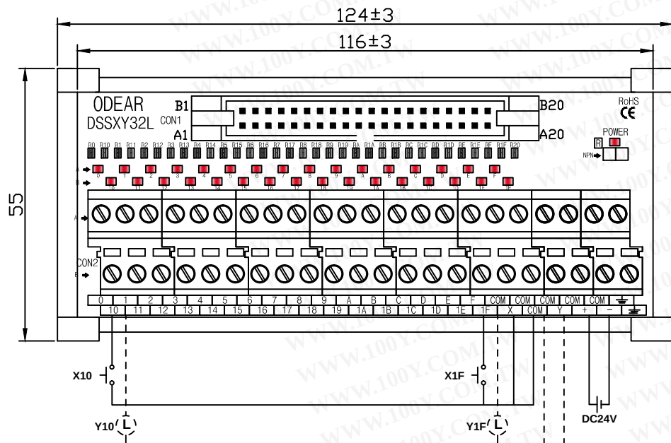
CONNECTOR 腳位定義
