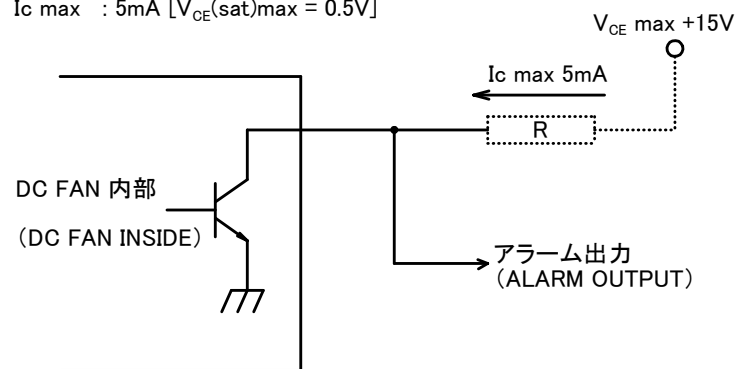
図1 アラーム信号回路 (ALARM SIGNAL CIRCUIT)
