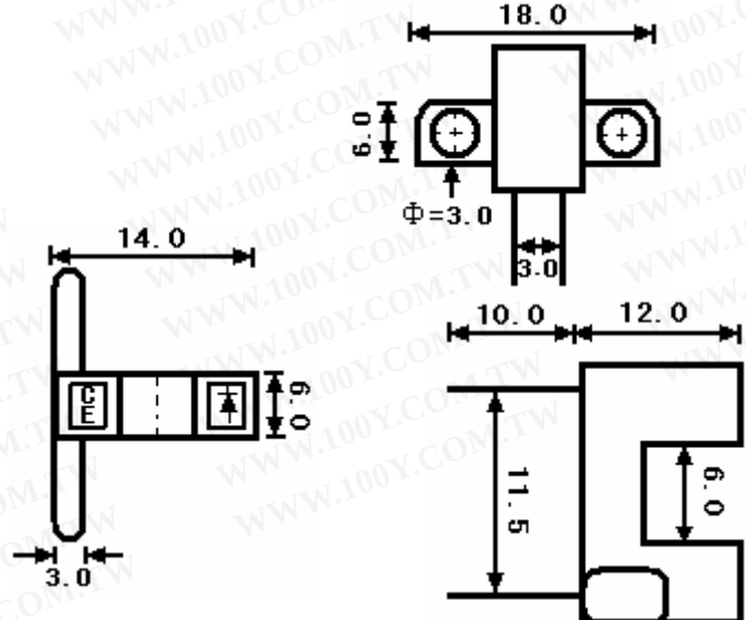
图6. 外形尺寸图 单位 (mm)
