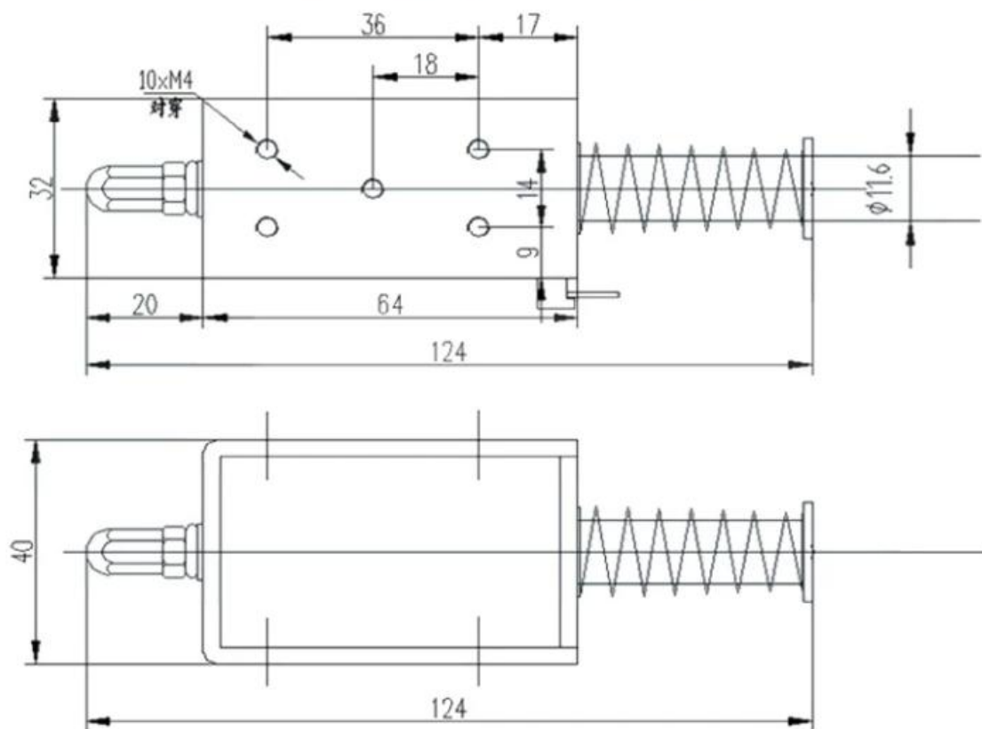
电磁铁外形尺寸图
