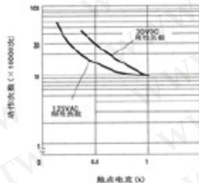
电气寿命曲线
