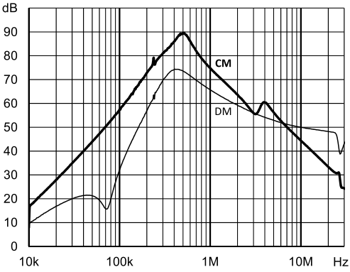
FN3287-40-33-C33-R65
