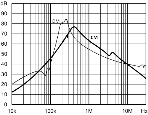
FN3287-125-35-C33-R65
