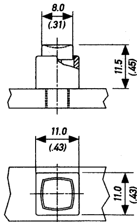
Square Button PBS Square Bezel BZS
