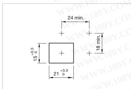
Einbauöffnungen [mm]
