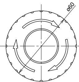
ø60mm特大蘑菇头形按钮
