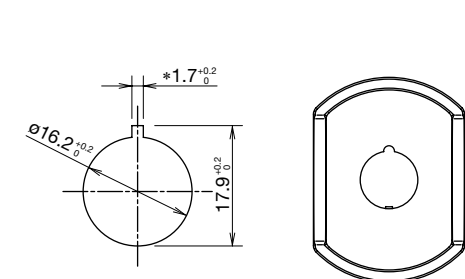
φ16mm 紧急遮断用开关保护罩
