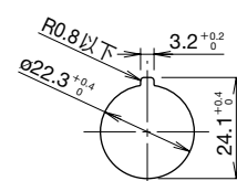
安装孔加工图
