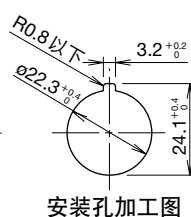
安装孔加工图
