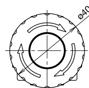
ø40mm大蘑菇头形按钮
