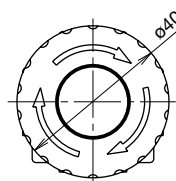
ø40mm 大蘑菇头形按钮
