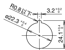
安装孔加工图
