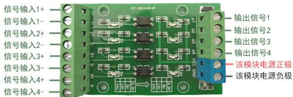
输入输出真值表(5V转24V)
