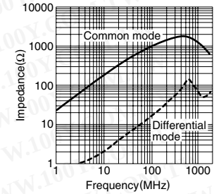
ACM3225-102-2P
