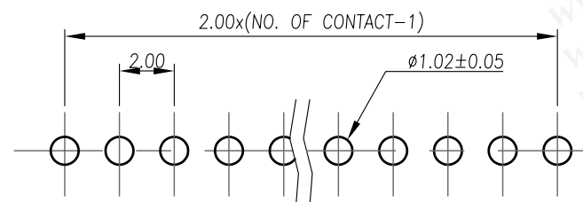
P.C.B. LAYOUT
