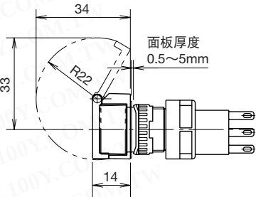
开关保护罩安装图
