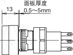
防尘罩安装图
