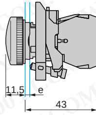
直接供电 XB4-BV6
