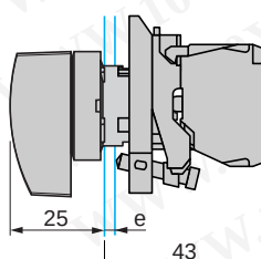
拨动开关头 ZB4-BD*8
