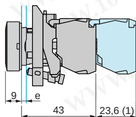
按钮，弹簧返回 XB4-BA**
