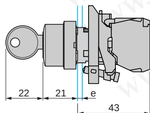
钥匙开关 XB4-BG
