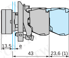
带指示灯双头按钮 带 LED XB4-BW84•5
