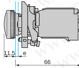
带小型变压器 XB4-BV3•, BV4•
