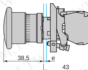
蘑菇头按钮，弹簧返回 XB4-BC21
