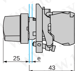
钥匙开关 XB4-BG
