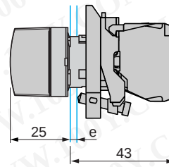
带指示灯选择开关 带 LED XB4-BK12••5
