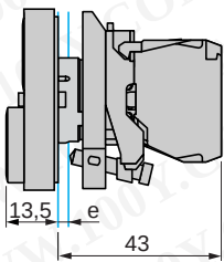
e : 带指示灯双头按钮 1 - 6 mm.
