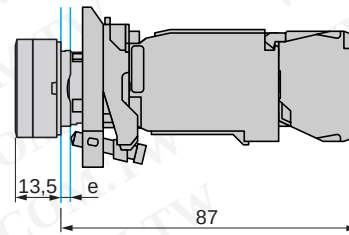
带指示灯选择开关 带 LED XB4-BK12••5
