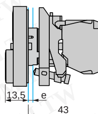
双头按钮，弹簧返回 XB4-BL*45, BL*4C5
