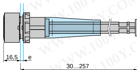
手动过载复位按钮 XB4-BA9••
