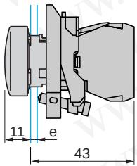
带指示灯 带 LED XB4-BVB•, BVG•, BVM•
