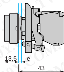
XB4-BL**
