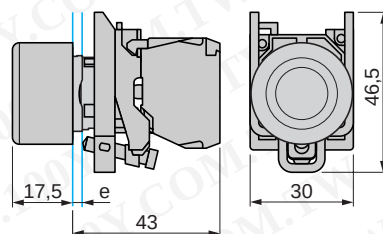
XB4-BP**
